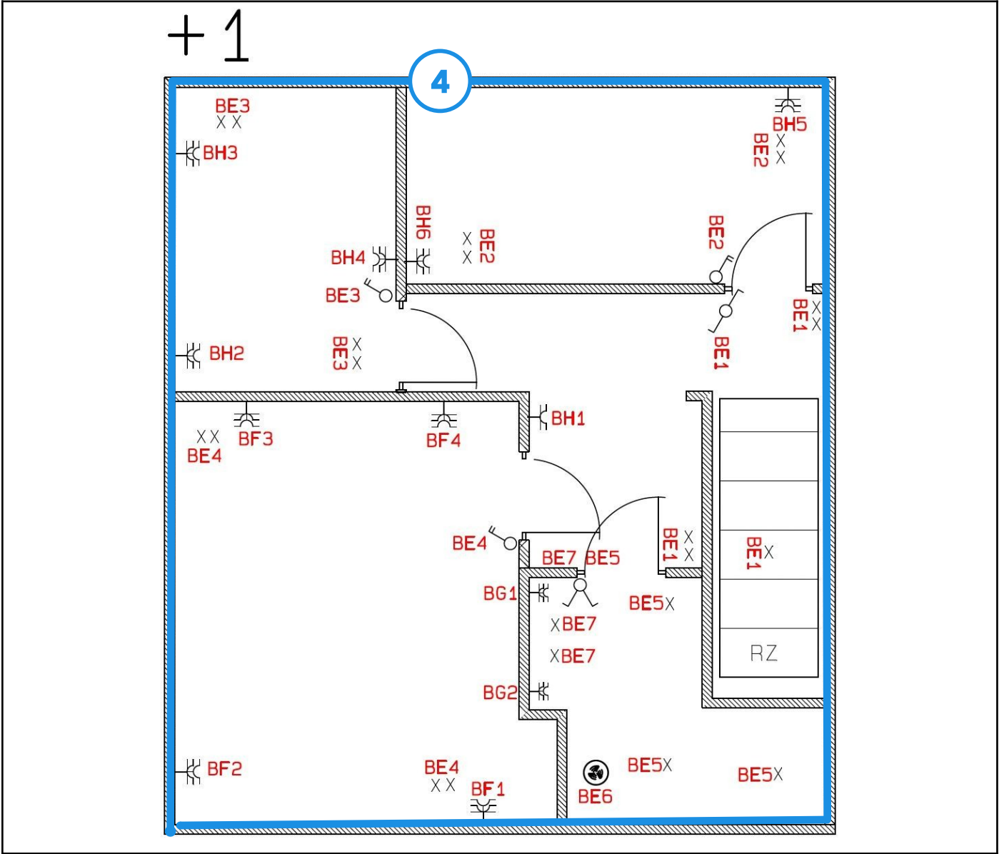
Legende van plan 1.2: Schets eerste verdiep
