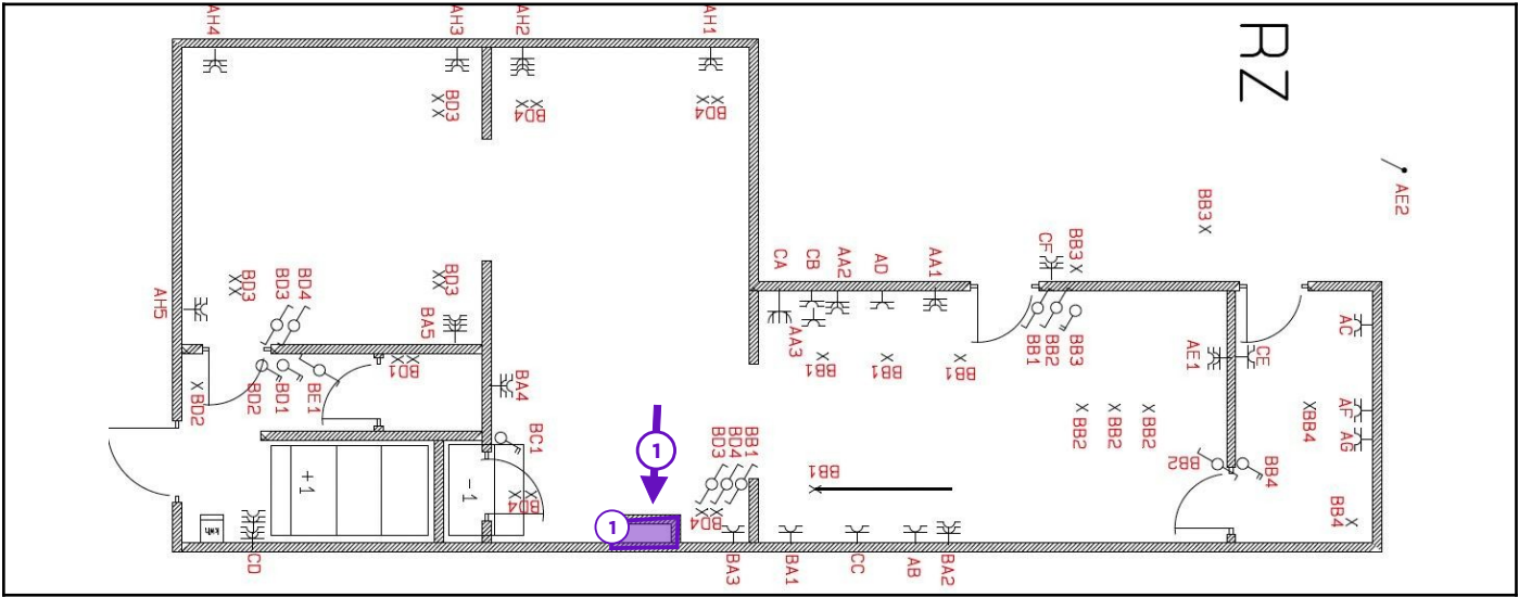
Legende van plan 1.5: Schets gelijkvloers
